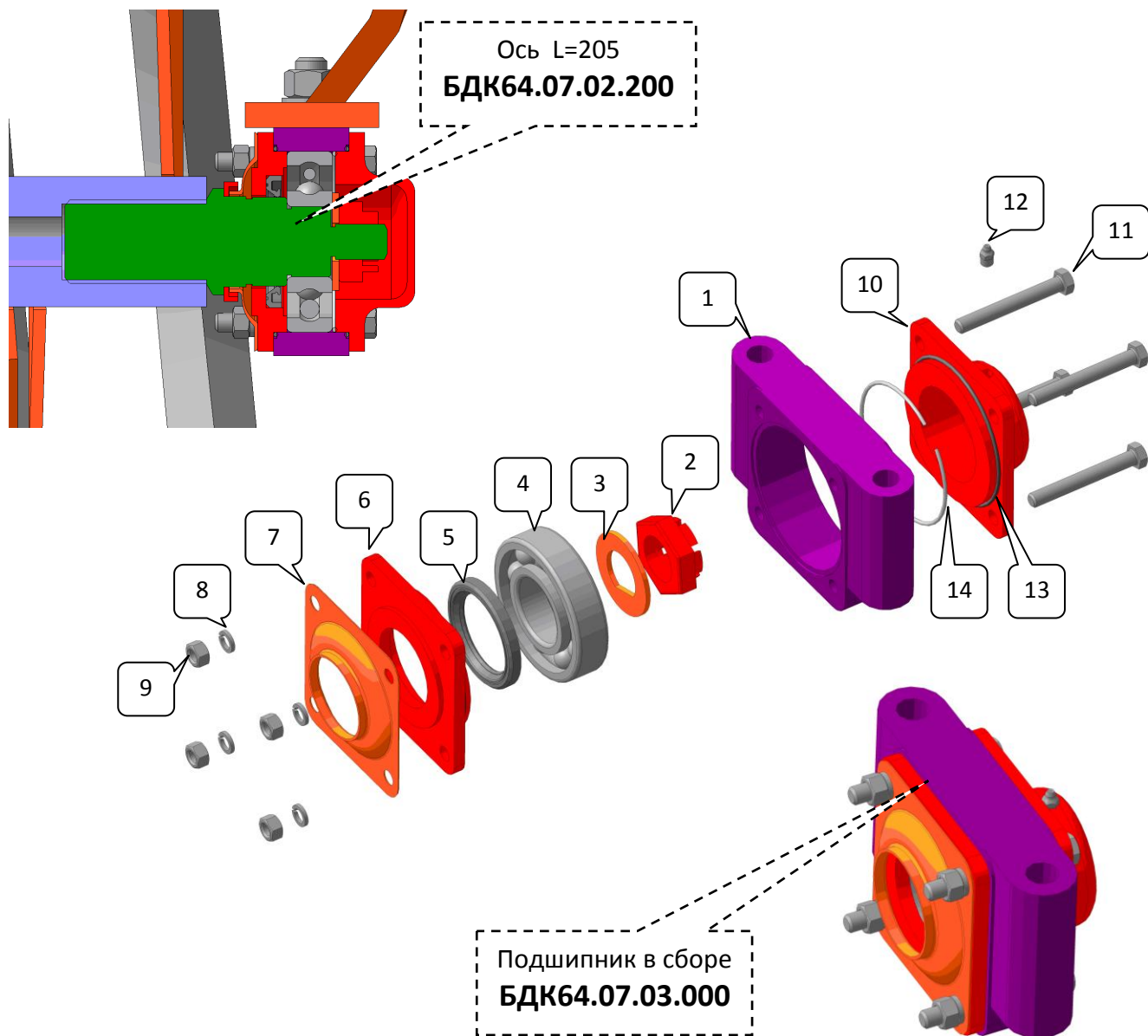
Подшипник катка в сборе БДК64.07.03.000
