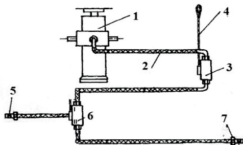
Рис. 1 Схема гидравлической системы механизма опрокидывания грузового кузова 1 – гидроцилиндр, 2 – гидравлические шланги, 3 – запорный клапан, 4 – трос, управляющий запорным клапаном, 5 – наконечник соединительного клапана, 6 – управляющий клапан, 7 – гнездо соединительного клапана.
