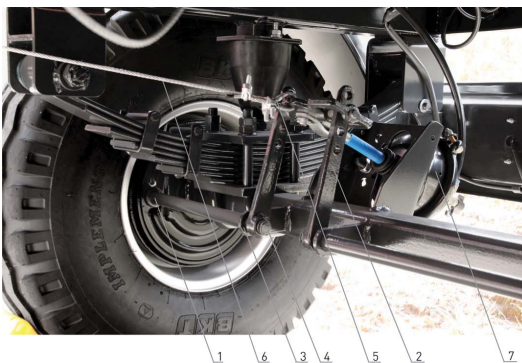
Рис. 6. Элементы тормозной системы: 1 – вал тормозного кулака, 2 – рычаг (плечо) вала тормозного кулака, 3 – регулирующий „гребень” на вале тормозного кулака, 4 – гайка, регулирующая положение рычага на вале, 5 – тяга (толкатель), соединяющая поршень пневмоцилиндра с плечом вала тормозного кулака, 6 – трос стояночного тормоза, 7. – мембранный пневмоцилиндр.
